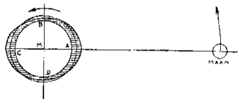
Figuur 1. De eb- en vloedbeweging der zee onder invloed van aantrekkende werking der maan.
